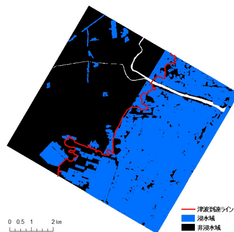
図2 浸水域抽出結果 (赤：国土地理院が公開した津波浸水ライン、青：提案手法による浸水域抽出結果)
